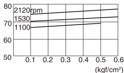
dB(A) SSR-100
