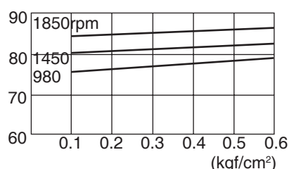
dB(A) SSR-200H
