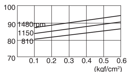
dB(A) SSR-200H
