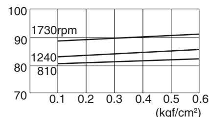
dB(A) SSR-150
