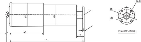
Suction Silencer (KSE)
