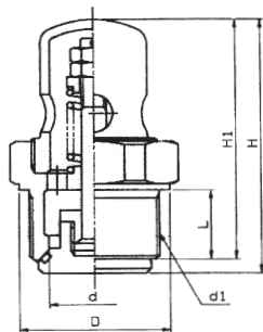
Suction Silencer (KSE)
