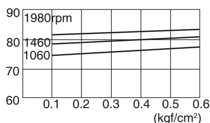
dB(A) SSR-175
