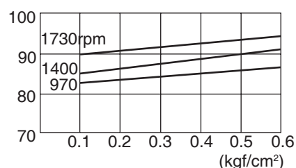
dB(A) SSR-175
